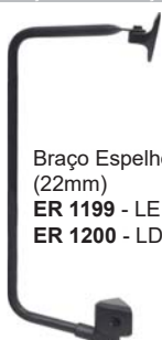
Conjunto Espelho Retrovisor - LE Nº Compatível 9798101216/7316 ER 177 - sem Desembaçador Convexo 01 PÇ ER1196, 01 PÇ ER1199 ER 179 - com Desembaçador Convexo 01 PÇ ER1197, 01 PÇ ER1199 ER 181 - com Desembaçador Convexo - Elétrico (24V) 01 PÇ ER1198, 01 PÇ ER1199
