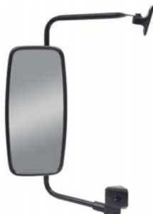
Conjunto Espelho Retrovisor - LE Nº Compatível 9798102316 ER 183 - sem Desembaçador Plano 01 PÇ ER1062, 01 PÇ ER1201 ER 185 - sem Desembaçador Convexo 01 PÇ ER1063, 01 PÇ ER1201
