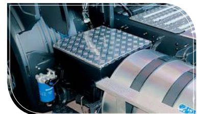
EC 068 Protetor Alumínio Caixa Bateria SC R 114/124 / P/G/R Highline até 2015 (FT 163)
