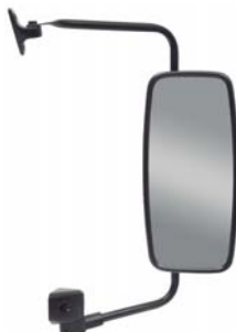
Conjunto Espelho Retrovisor - LD Nº Compatível 9798102416 ER 184 - sem Desembaçador Plano 01 PÇ ER1062, 01 PÇ ER1202 ER 186 - sem Desembaçador Convexo 01 PÇ ER1063, 01 PÇ ER1202
