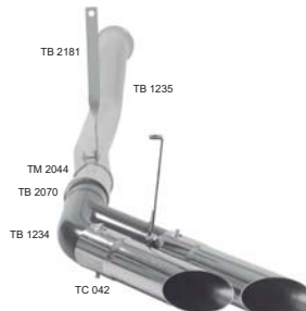
TB 150 - Volvo FH 2021 - LE
